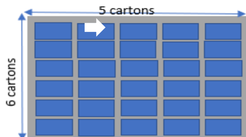
Disposition sur la palette US (vue du dessus) sur 7 couches
