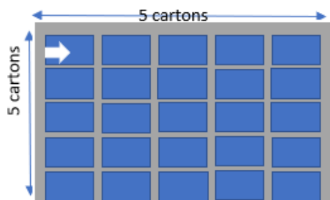
Disposition sur la palette Europe (vue du dessus) sur 7 couches
