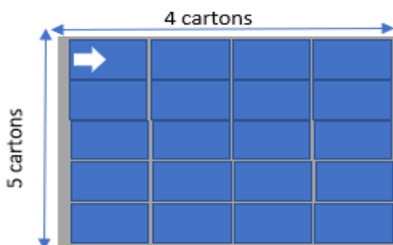
Disposition sur la palette US (vue du dessus) sur 5 couches
